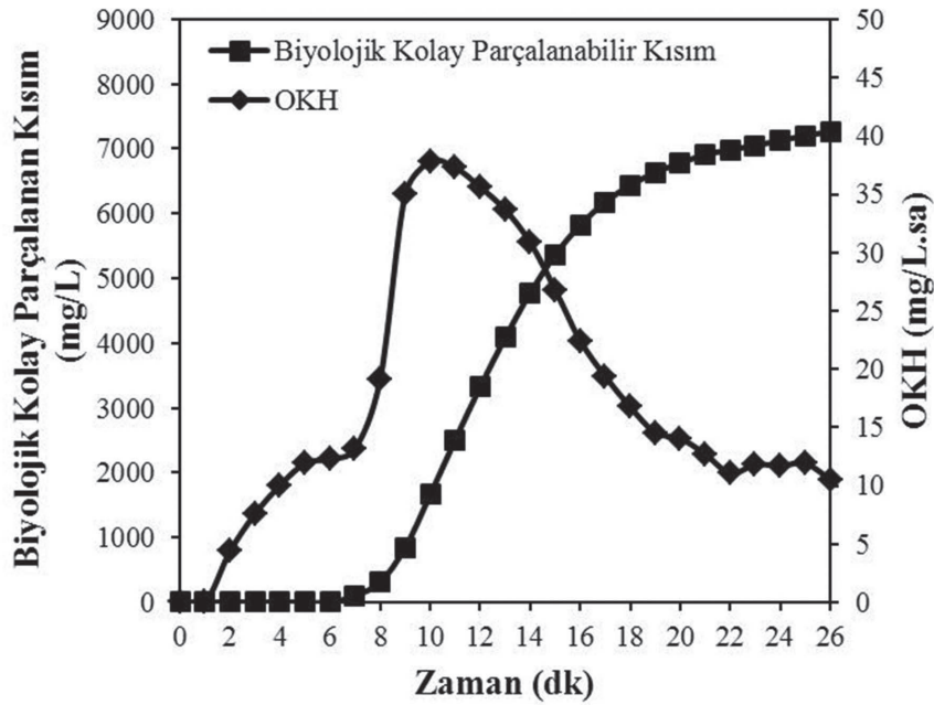
Şekil 2. Respirometrik olarak zeytin karasuyunda mikroorganizmaların OKH'leri nin değişimi ve kolay parçalanabilir BOİ değerinin değişimi
