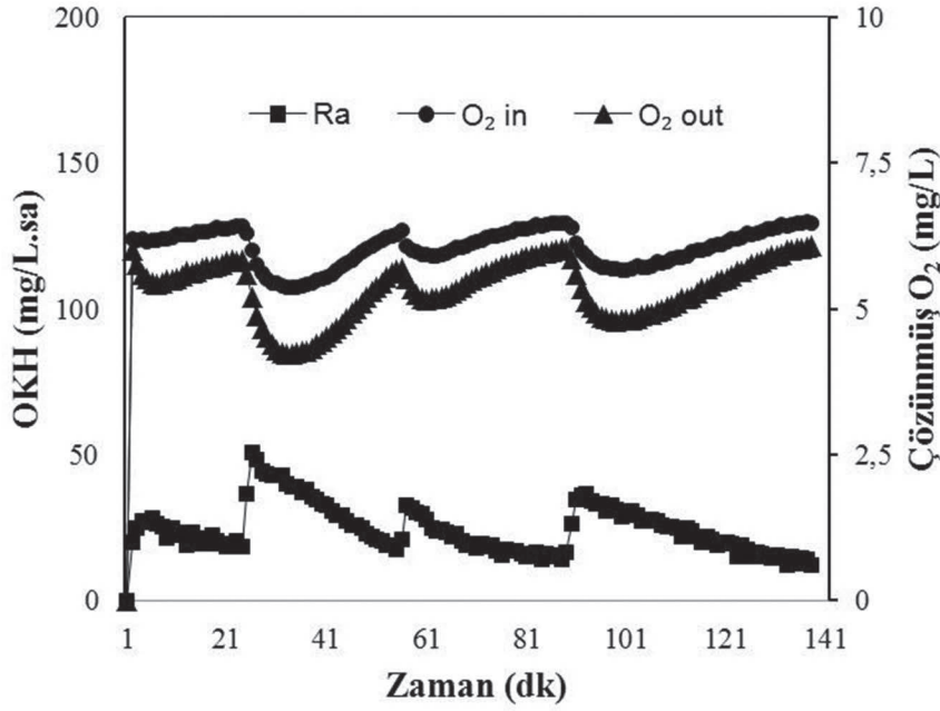
Şekil 3. Respirometrik olarak zeytin karasuyunda Ra ve çözünmüş oksijen değişimi
