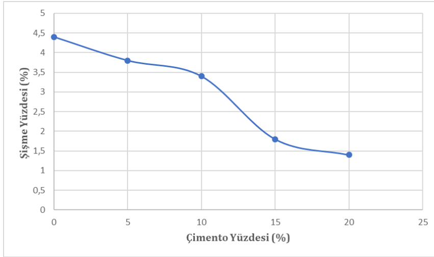
Şekil 11. Çimento yüzdesine bağlı numune şişme yüzdesi değerlerinin grafikte gösterimi
