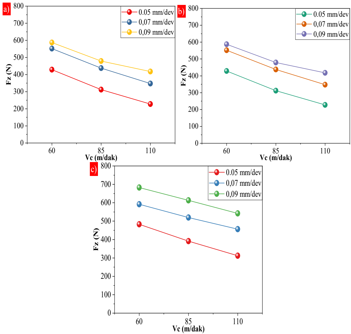
Şekil 3. Monel 400 süper alaşımasının tornalanmasında ölçülen esas kesme kuvveti; a) a_p=0,4 mm, b) a_p=0,8 mm ve c) a_p=1,2 mm
