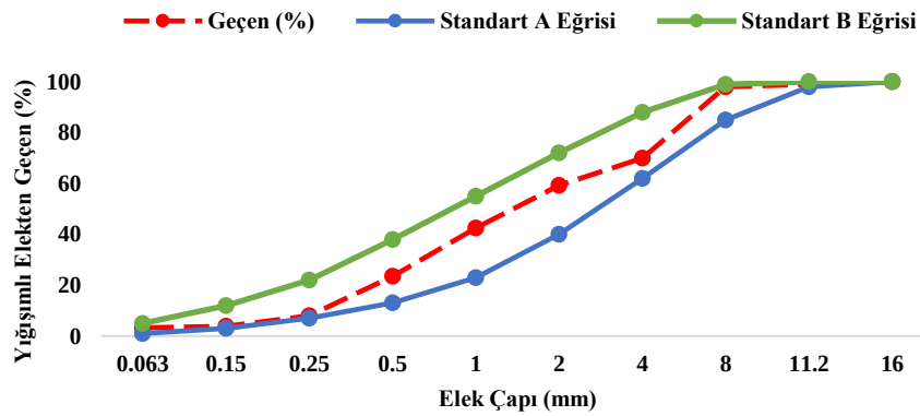
Şekil 1. Agregat granülometri eğrisi
