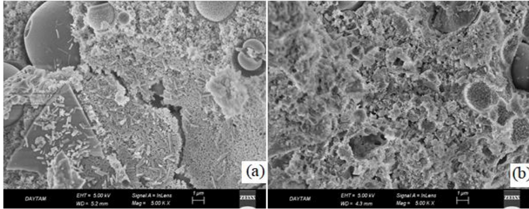
Şekil 8. U100 karışımının 200°C (a) ve 400°C (b) için SEM görüntüleri
